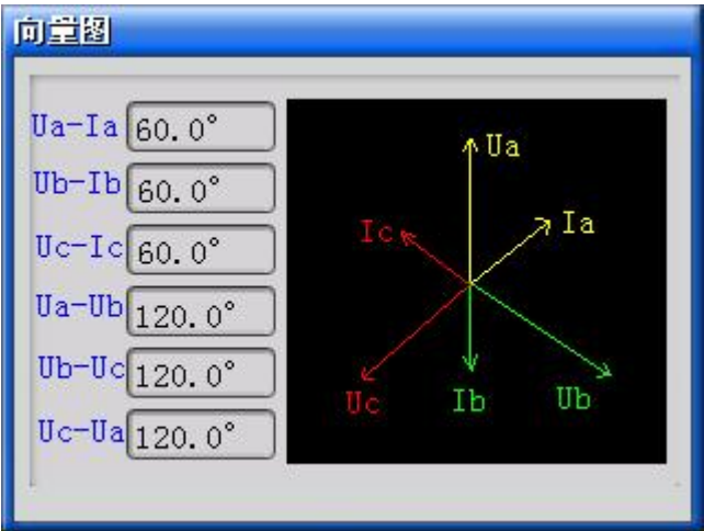
图8 向量图
