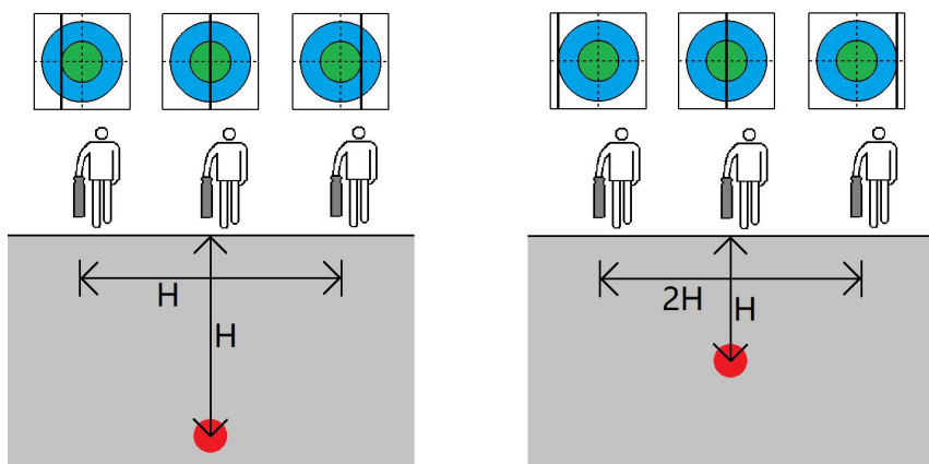
A.绿环相切，等于深度
