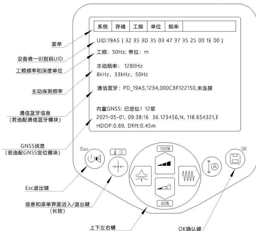
图 1-6-1 接收机信息和菜单界面示例
