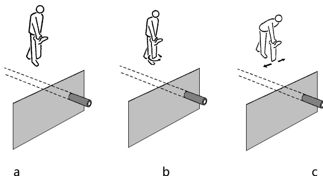
图 4-1-9 精确定位
