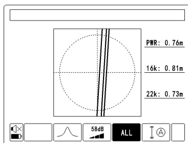
图 5-1-2 管线区分示例
