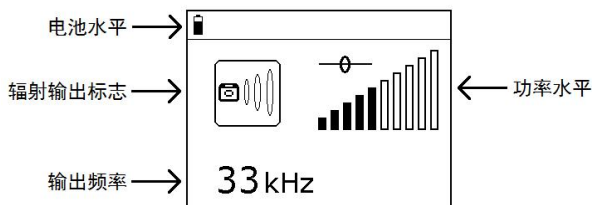
图 2-3-2 卡钳耦合输出界面显示
