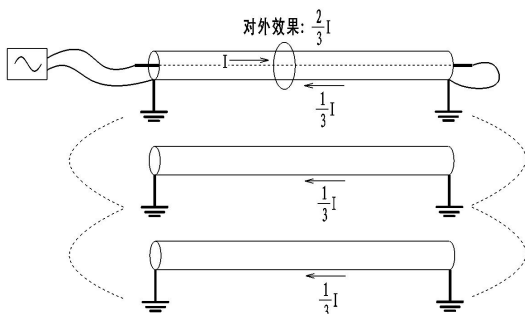
图 3-1-3 相线 - 护层接法
