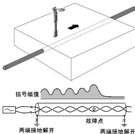
图 8-1-1 相间短路故障定点
