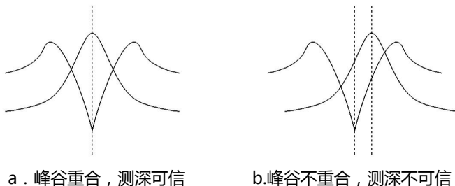
图 4-2-4 峰谷重合示例
