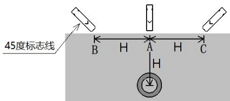
图 4-2-8 音谷 45°法测深
