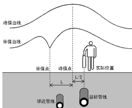
图 4-1-10 定位修正
