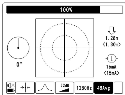
图 4-2-2 一键深度和电流测量
