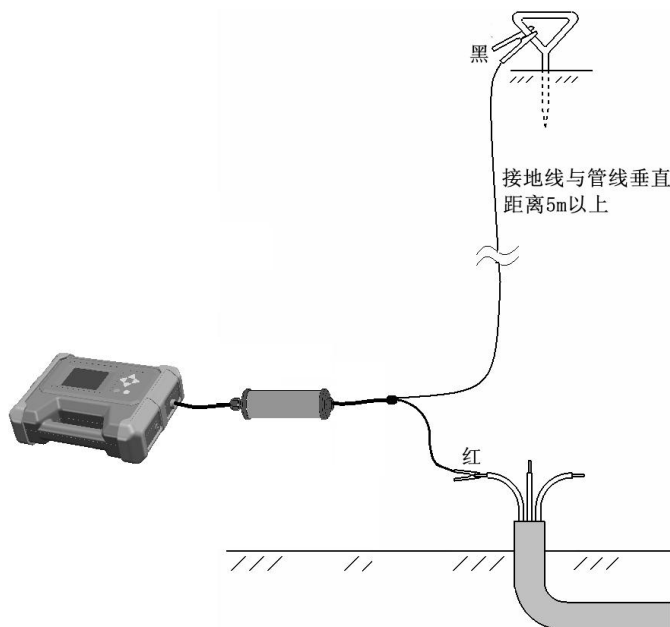
图 7-1-3 接地故障定点接线
