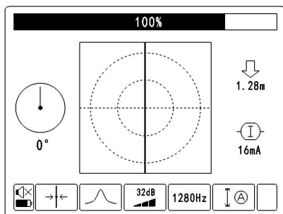
图 4-2-1 实时深度和电流测量
