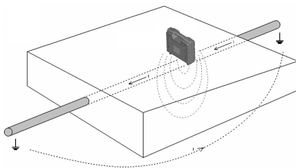
图 2-3-1 辐射感应法
