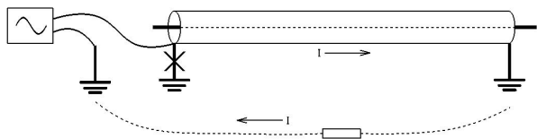
图 3-1-2 护层 - 大地接线法
