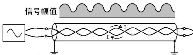
图 3-1-5 相间接法
