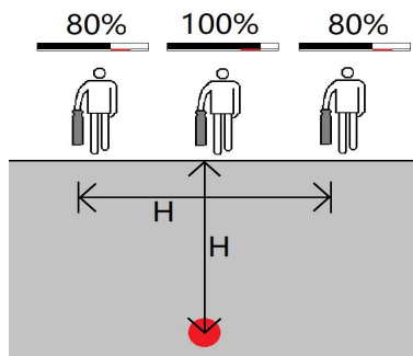
图 4-2-6 宽峰 80%法测深
