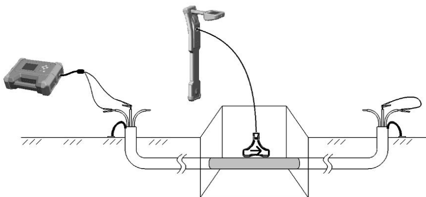
图 6-3-3 听诊器识别
