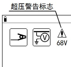
图 2-1-4 管线电压超压警告界面
