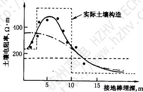
●●●● 测试数据 ——— 三层等值构造土壤的视在土壤电阻率计算曲线 - - - 两层等值构造土壤的视在土壤电阻率计算曲线 ..... 单层等值构造土壤的视在土壤电阻率计算曲线
