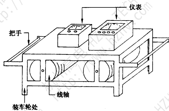
图 21 测试小车
