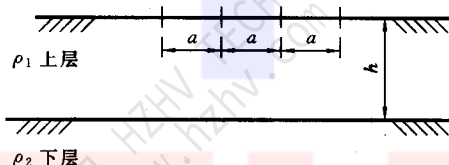
图 A1 两层土壤
