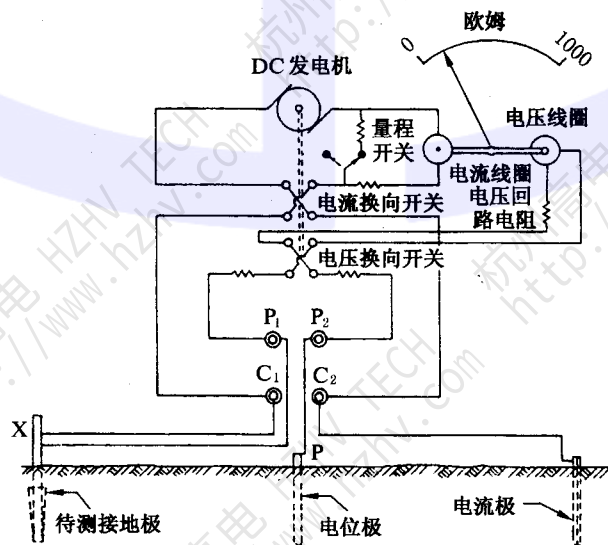
图 14 比率欧姆表
