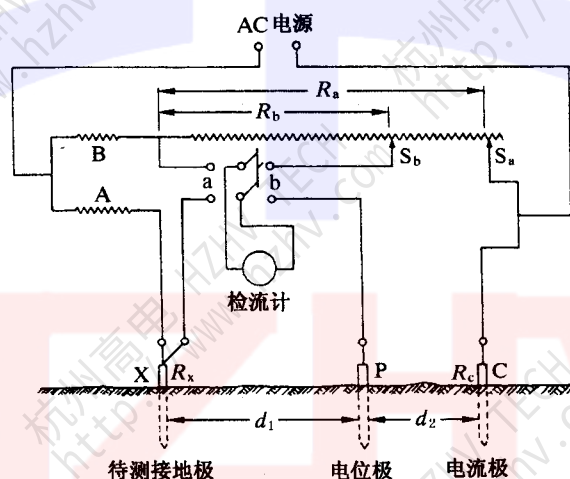
图 15 双平衡电桥
