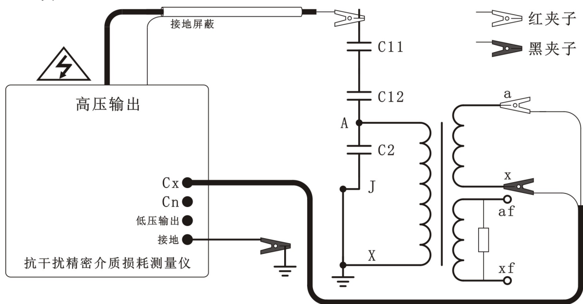
仪器高压线的芯线（红夹子）接 CVT 的上端，母线拆地，CVT 下端接地，低压线红、黑夹子接二次绕组。
