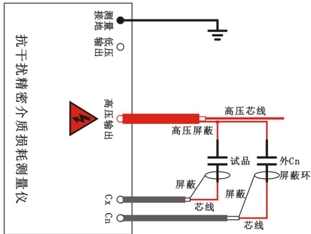
图 4-3 正接线、外标准电容、内高压（B、D、E、F、S、J 型有此功能）
