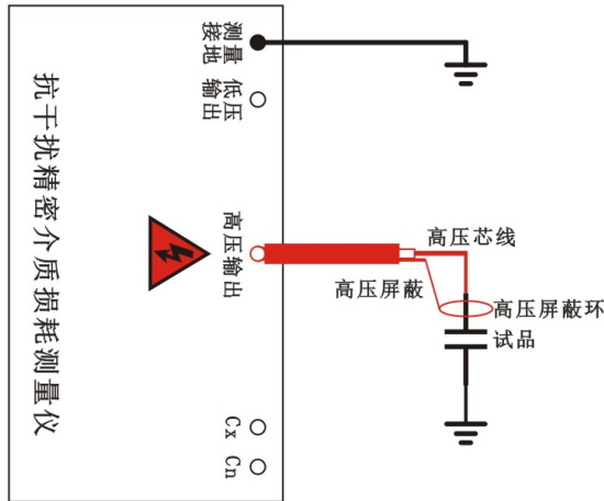
图 4-2 常规反接法参考接线图（B、D、E、F、S、J 型有此功能）
