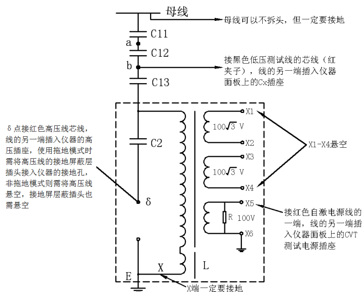
图 5-3 C13 和 C2 的测量方法（选择内标准、CVT 自激法、2kV 测试电压）
