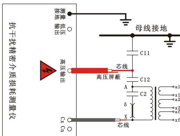
图 4-9 反接线低压屏蔽 (D、E、F、S、J 型有此功能)
