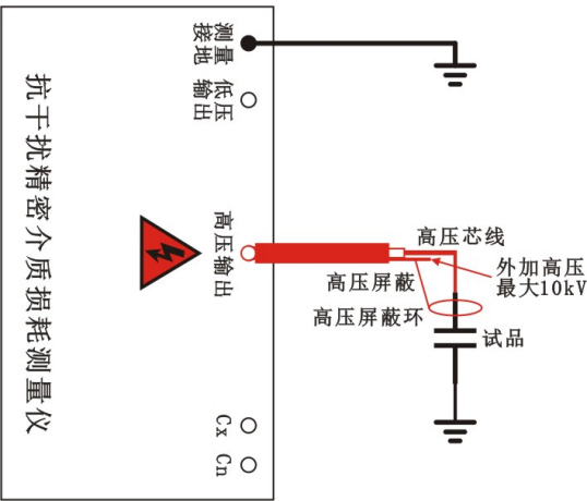
图 4-6 反接线、内标准电容、外高压（B、D、E、F、S、J 型有此功能）
