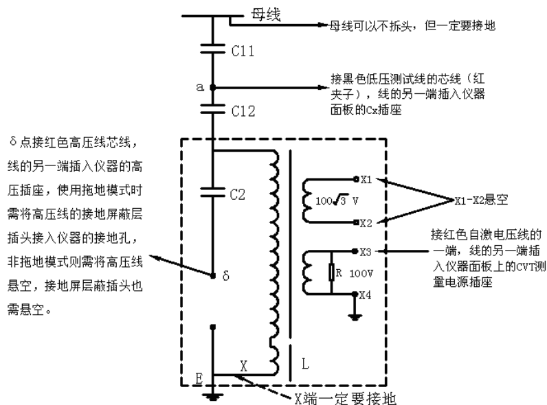
图 5-5 C12 和 C2 的测量方法（选择内标准、CVT 自激法、2kV 测试电压）
