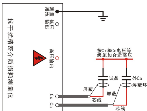
图 4-7 正接线、外标准电容、外高压（高电压介损，B、D、E、F、S、J 型有此功能）
