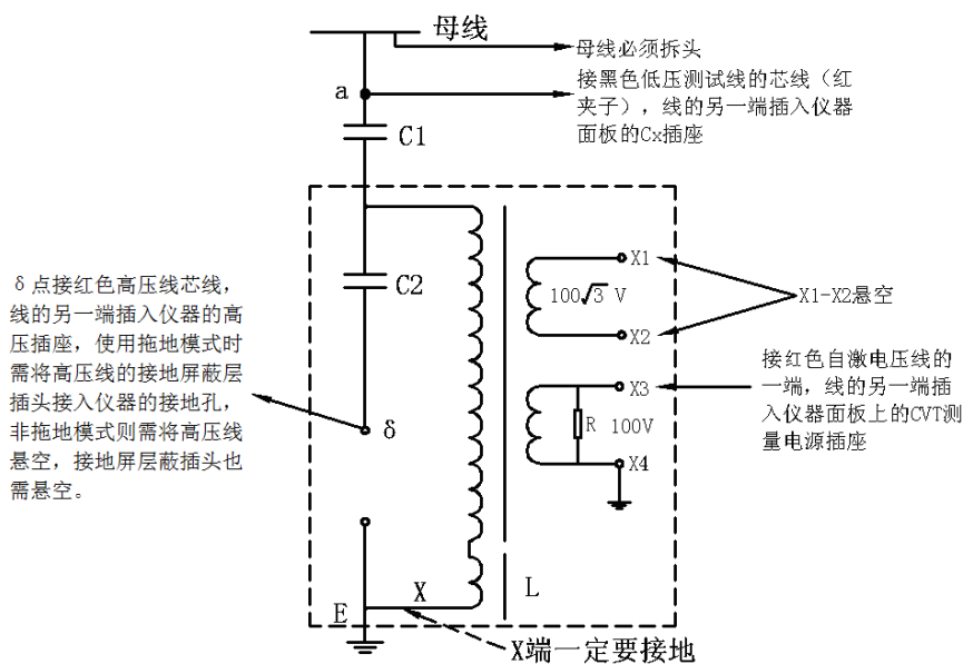
图 5-6 C1 和 C2 的测量方法（选择内标准、CVT 自激法、2kV 测试电压）
