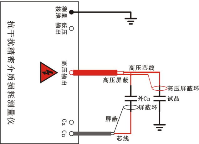
图 4-4 反接线、外标准电容、内高压（B、D、E、F、S、J 型有此功能）
