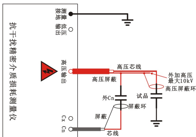
图 4-8 反接线、外标准电容、外高压 (B、D、E、F、S、J 型有此功能)
