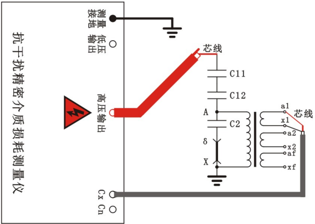
图 4-11 CVT 变比测试（E、F、S、J 型有此功能，CVT 二次侧电压需小于 120V）
