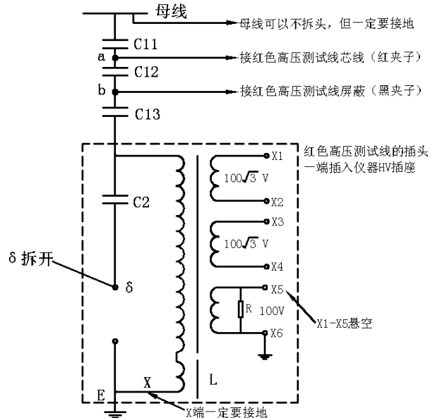
图 5-1 C11 的测量方法（选择内标准、反接线、10kV 测试电压）
