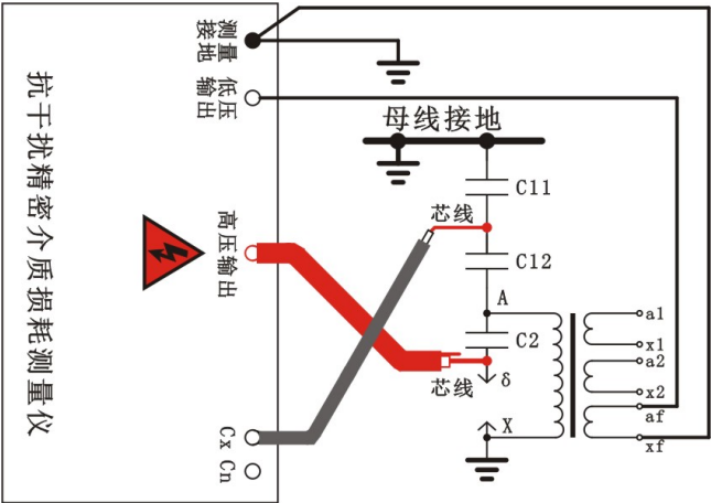
图 4-10 CVT 自激法（D、E、F、S、J 型有此功能）
