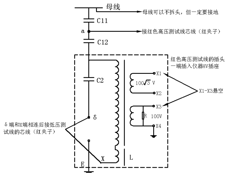
图 5-4 C11 的测量方法（选择内标准、反接线低压屏蔽、10kV 测试电压）
