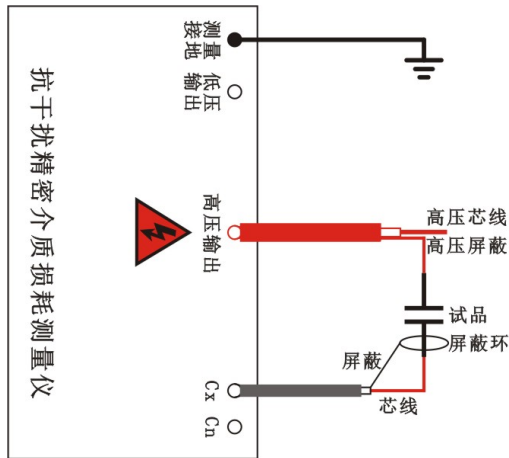
图 4-1 常规正接法参考接线图（B、D、E、F、S、J 型有此功能）
