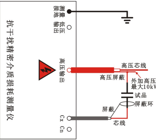
图 4-5 正接线、内标准电容、外高压（B、D、E、F、S、J 型有此功能）
