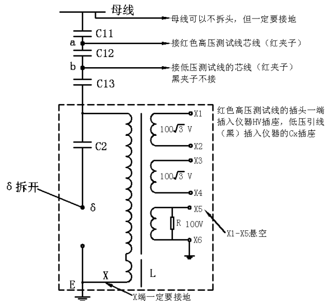
图 5-2 C12 的测量方法 (选择内标准、正接线、10kV 测试电压)
