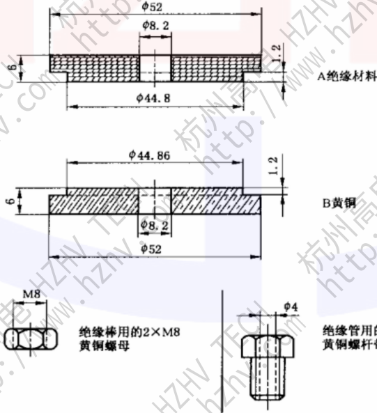
图 A.4 保护电极A、B部件结构图
