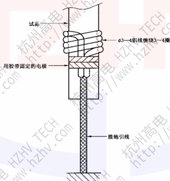
图 B.2 电极布置详图
