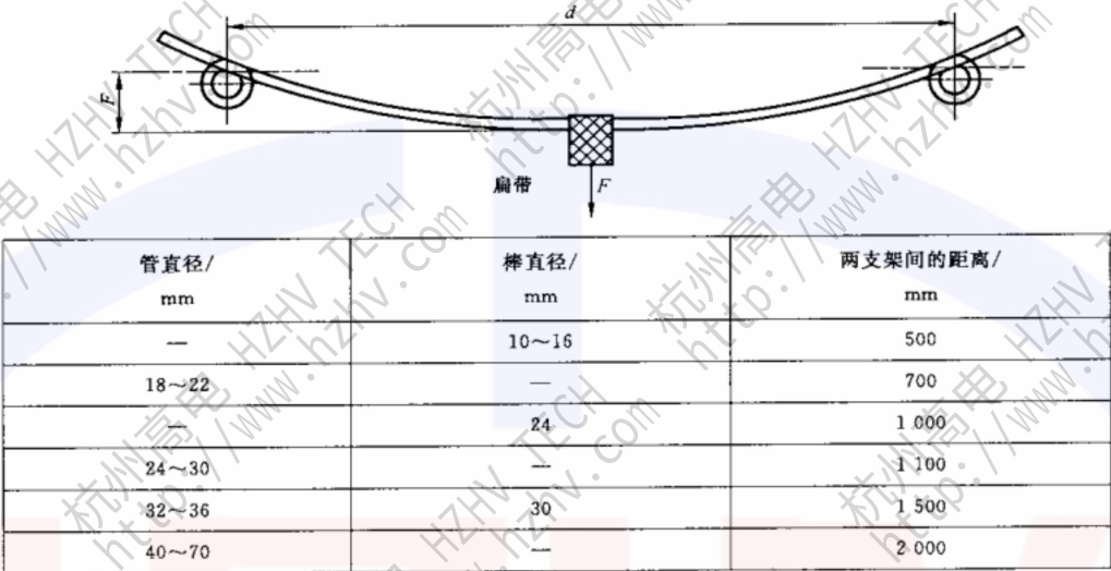
图 C.1 弯曲试验——试验装配图
