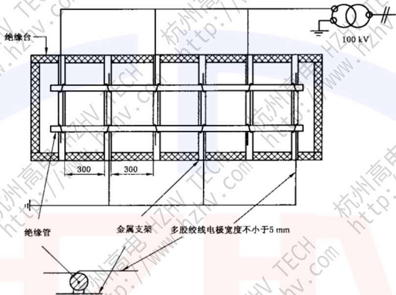
图 D.1 典型试验布置
