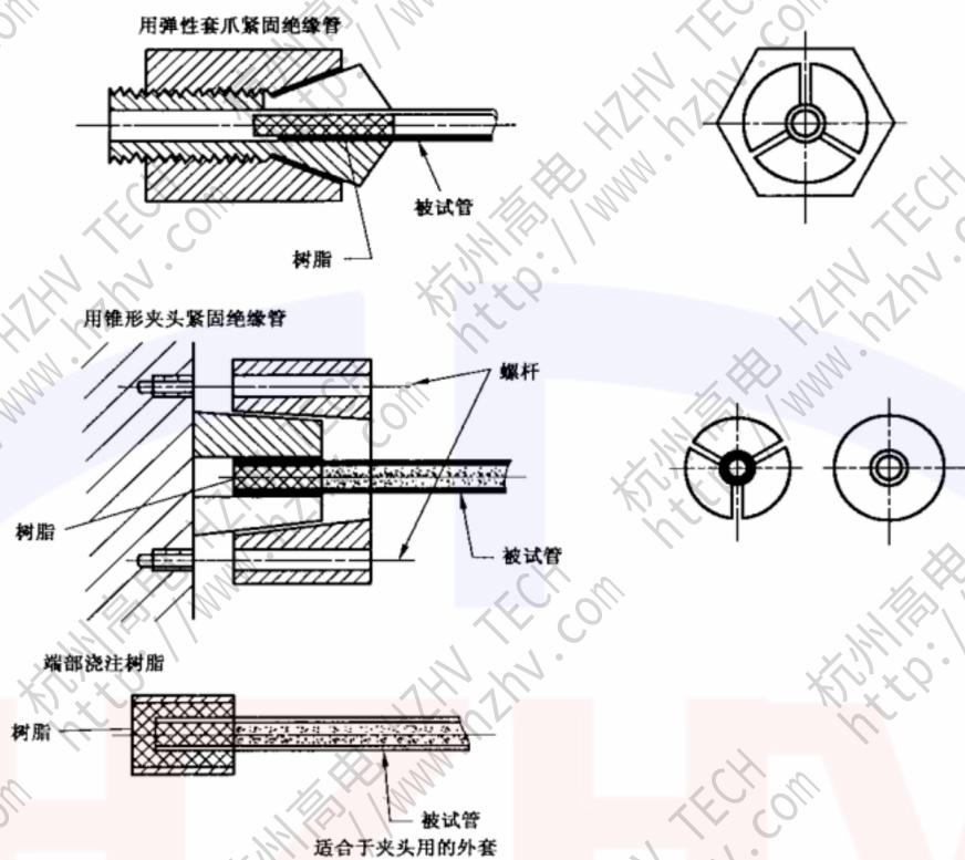
图 C.3 扭力试验——绝缘杆固定法示例
