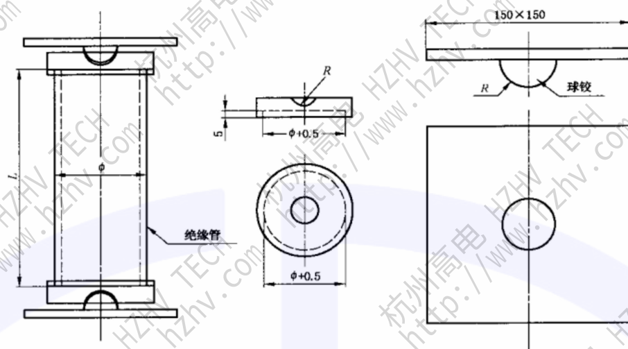
图 C.5 轴向压力试验——绝缘管固定示例
