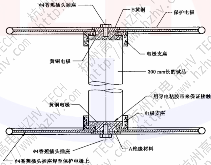
图 A.1 典型试验回路
