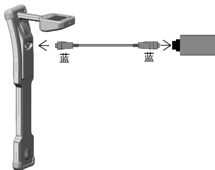
图 5-3-1 听诊器连接
