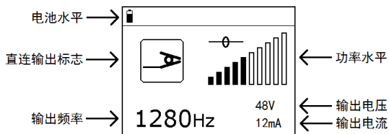
图 2-1-5 直连输出界面显示
