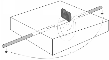
图 2-3-1 辐射感应法
