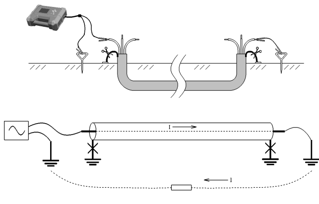
图 3-1-1 芯线 - 大地接线法
