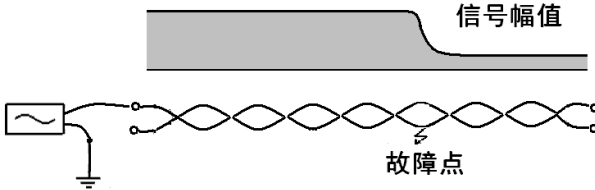
图 7-4-1 无铠装电缆相对地故障接线法
