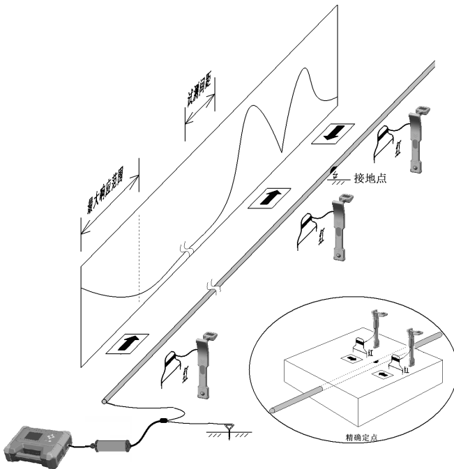
图 6-1-6 A 字架查障过程
