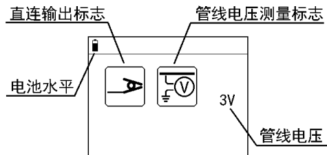
图 2-1-3 管线电压测量界面
