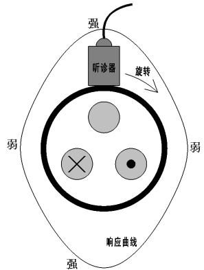
图 5-3-4 听诊器环绕测试
