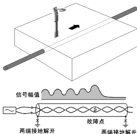
图 7-1-1 相间短路故障定点
