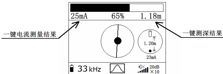
图 4-4-2 一键深度和电流测量
