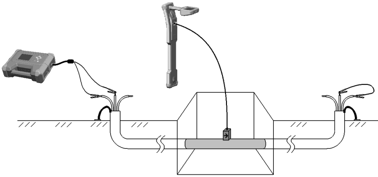
图 5-3-3 听诊器鉴别
