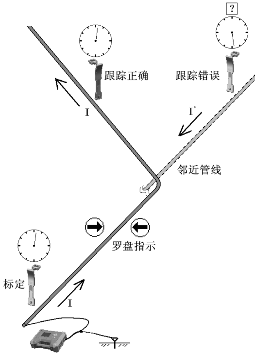
图 4-1-6 智能跟踪过程
