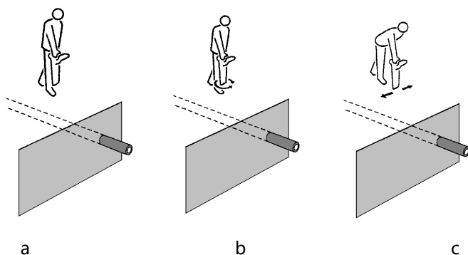
图 4-3-1 精确定位
