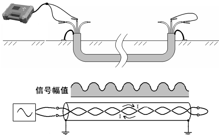
图 3-1-5 相间接法
