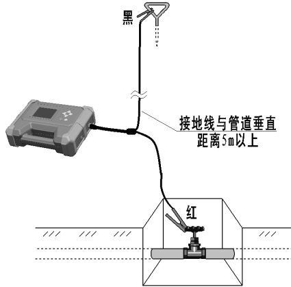
图 2-1-2 直连法接线
