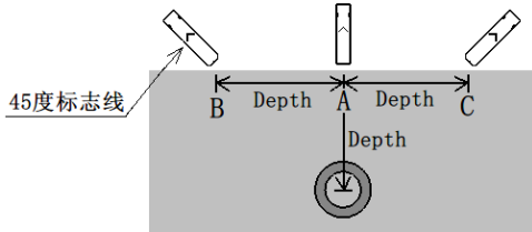
图 4-4-3 音谷 45°法测深
