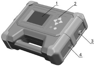
图 1-4-1 发射机整体
