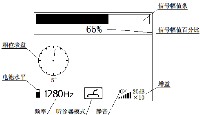
图 5-3-2 听诊器界面
