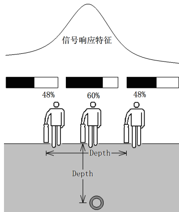
图 4-4-4 宽峰 80%法测深
