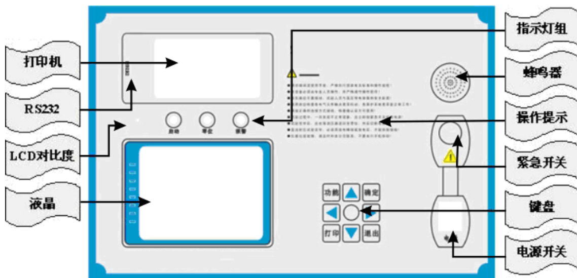
图 2 面板结构图
