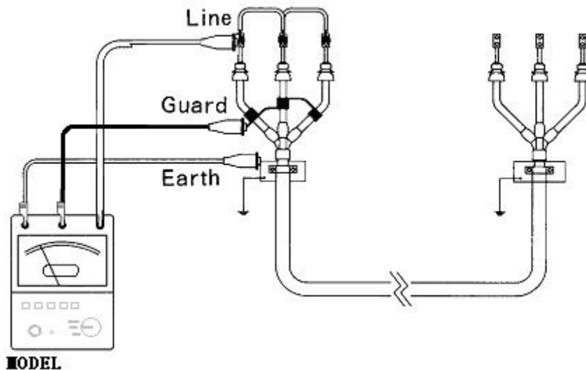
电缆芯对表皮绝缘测试图示
