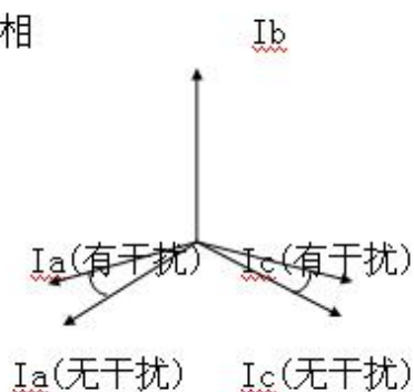
图十二 AC相受B相影响
