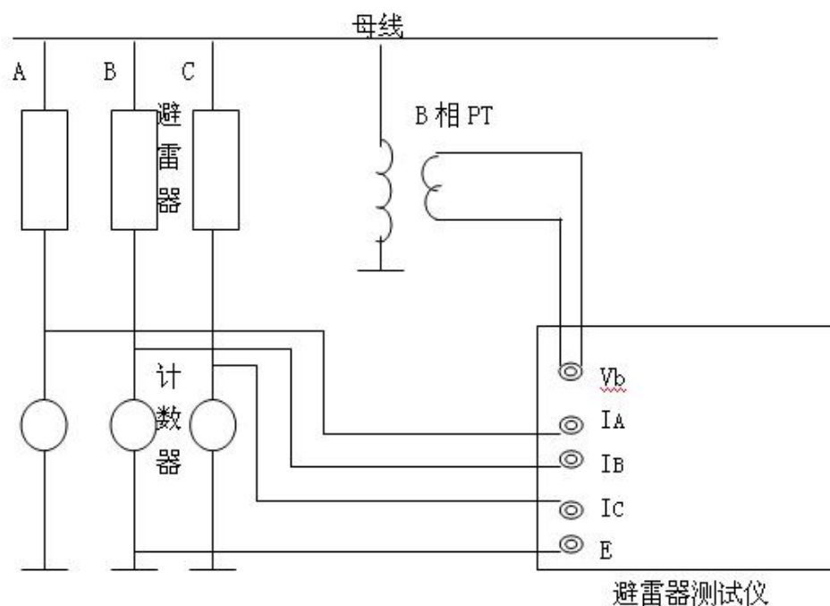
(图五) 三项同测
