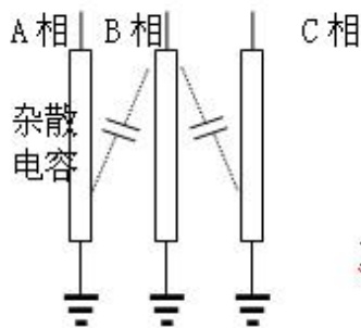
图十一 一字排列避雷器
