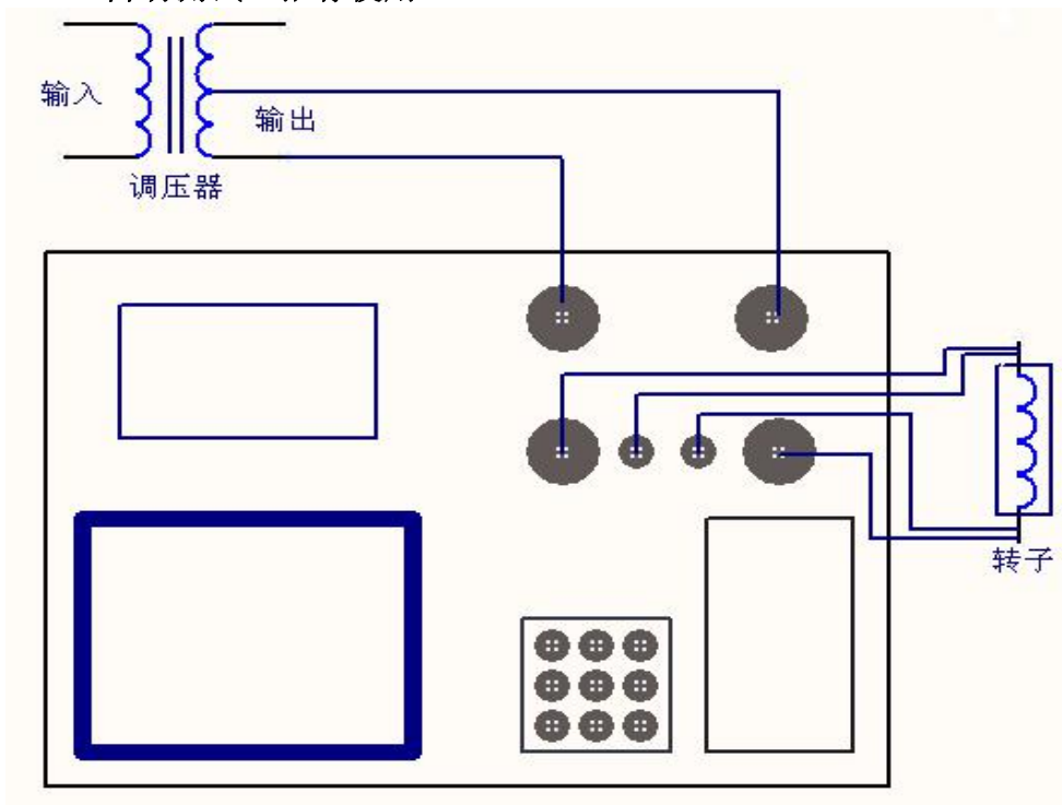
图 2. 转子交流阻抗试验接线图
