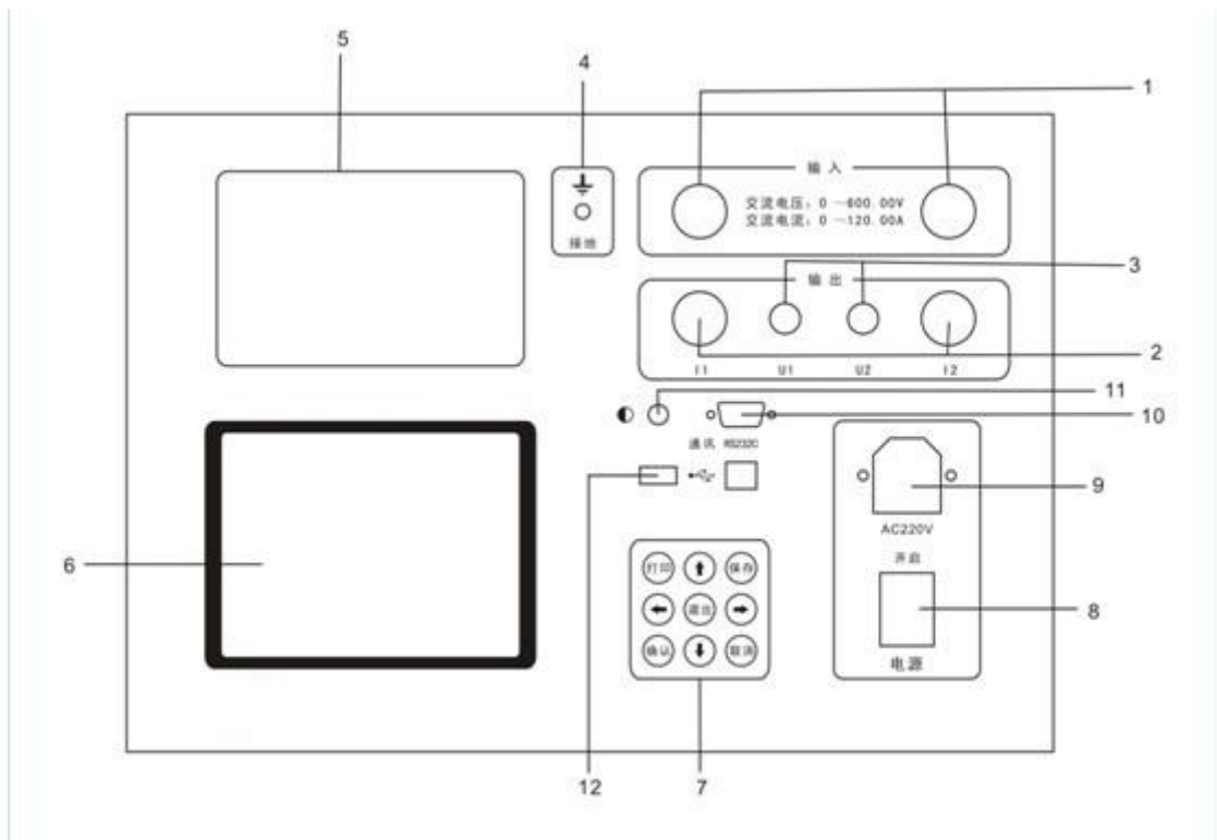
图 1. 面板结构图
