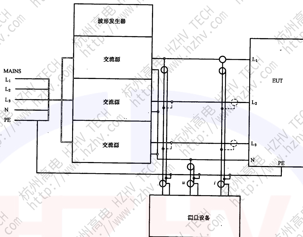
图 3 三相 EUT 试验布置举例
