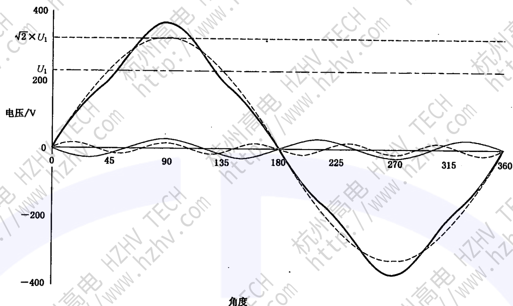
图 7 尖顶波波形
