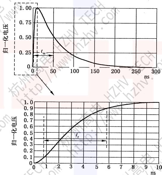
图 3 输出到 50 Ω 负载的单个脉冲的理想波形( t_r=5\text{ ns} , t_w=50\text{ ns} )
