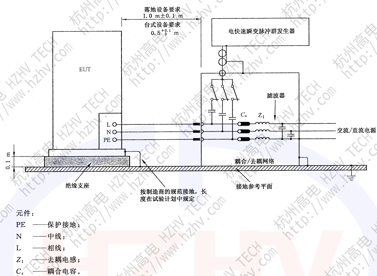
图 14 对交流/直流电源端直接耦合试验电压的实验室型式试验布置示例
