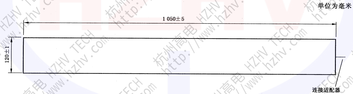
图 7 用于耦合夹校准的感应板
