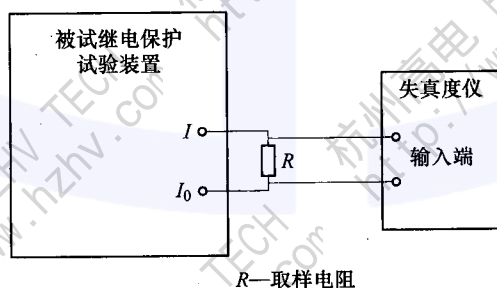
图 3 交流电流总谐波畸变率测量接线图
