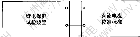
图 7 直流电流校准接线示意图
