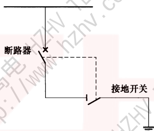
图 1 接地开关和断路器组合的例子
