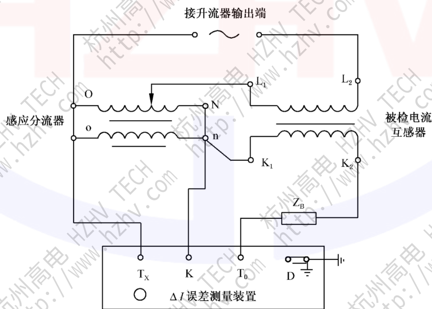
图 6 感应分流器检定电流互感器线路
