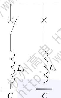
Figure H.1 – Diagramme du circuit de l'exemple 1
