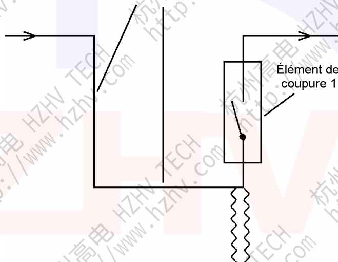
Figure 24 – Montage d'essai équivalent pour les essais sur éléments séparés d'un disjoncteur ayant plus d'un élément de coupure
