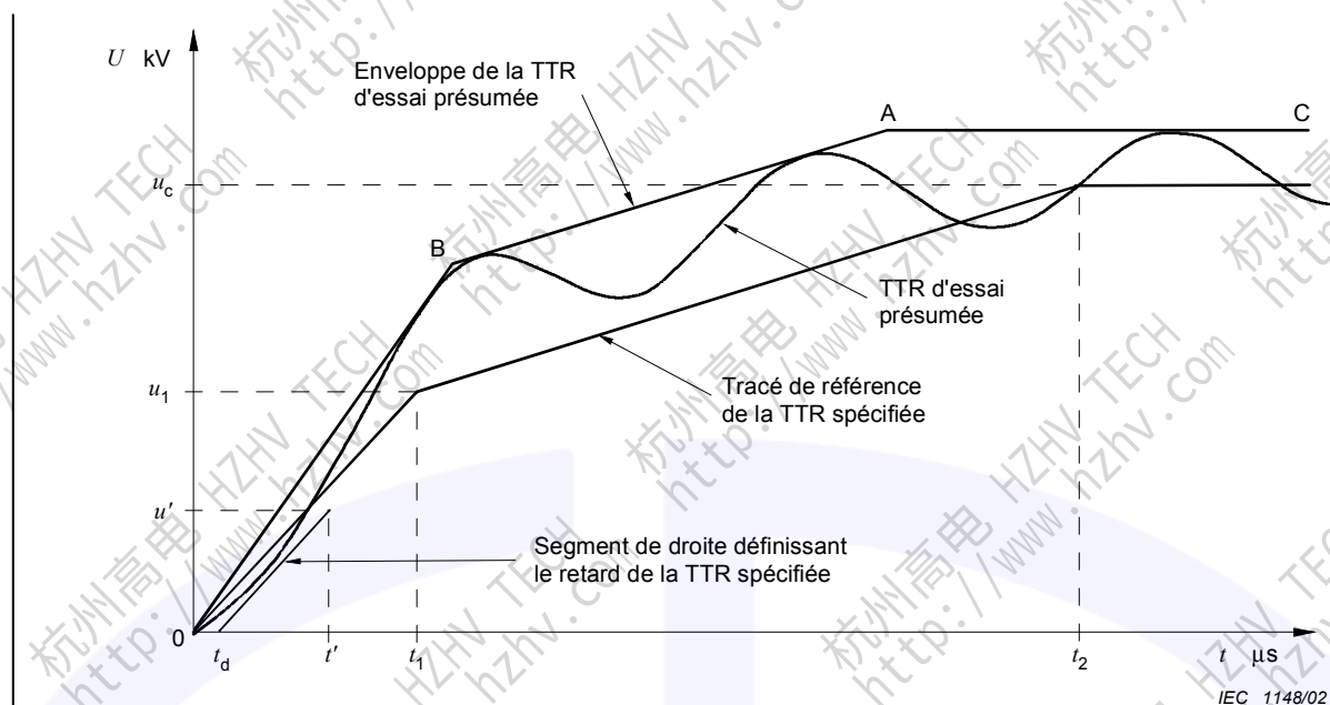
Figure 39 – Exemple d'une TTR d'essai présumée comportant une enveloppe à quatre paramètres et répondant aux conditions imposées pour l'essai de type – Cas de la TTR spécifiée comportant un tracé de référence à quatre paramètres
