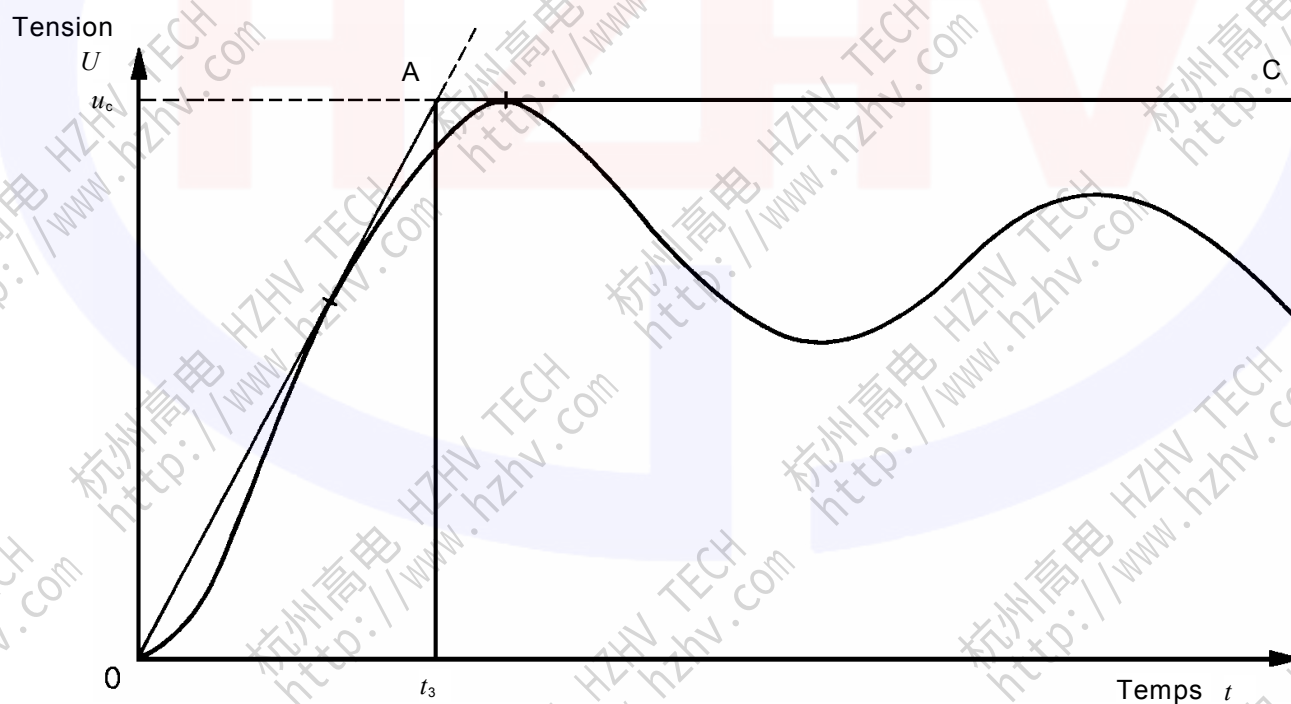
Figure E.4 – Représentation par deux paramètres d'une tension transitoire de rétablissement présumée d'un circuit – Cas du paragraphe E.2. c) 3) ii)
