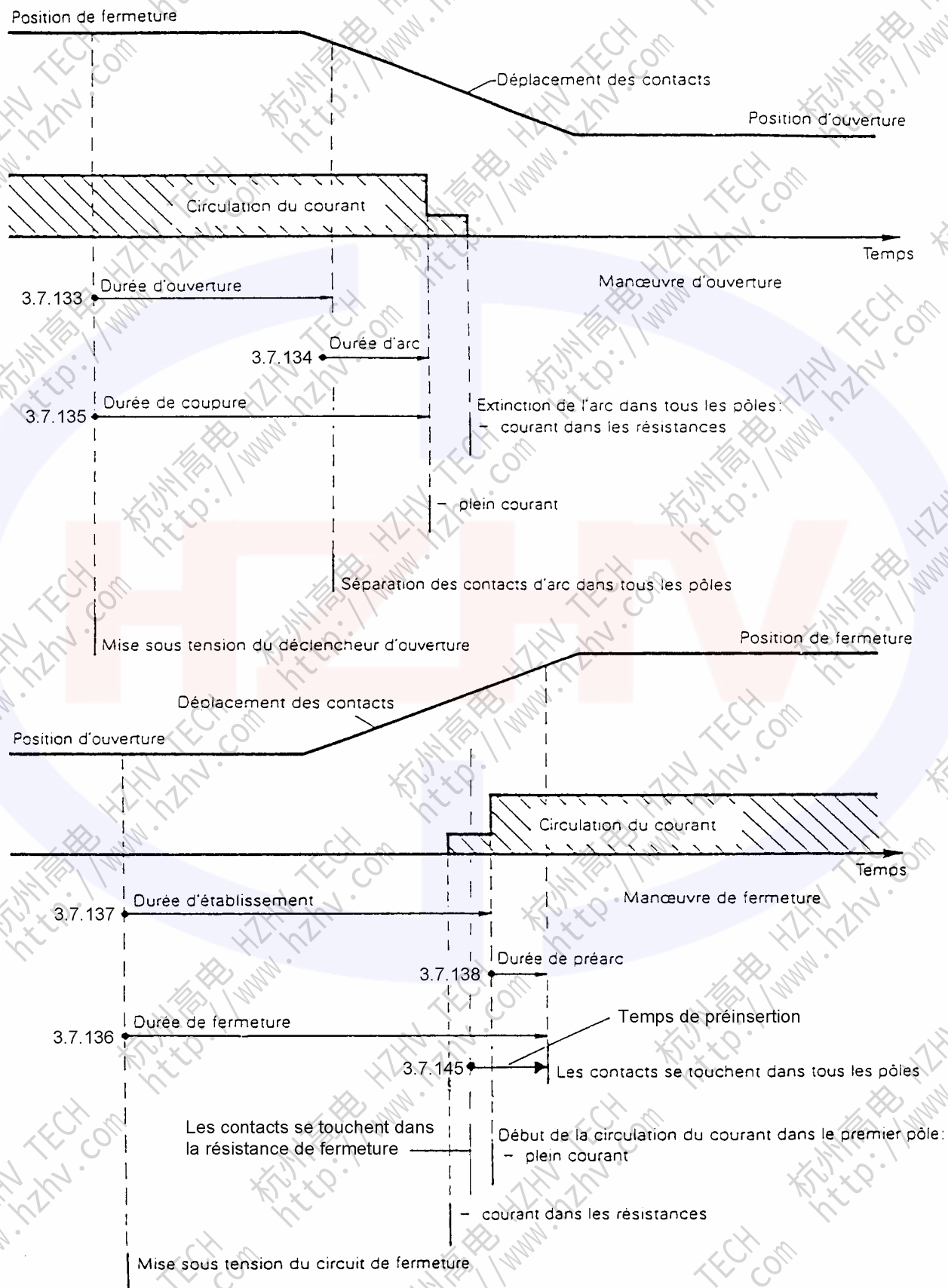
Figure 5 – Disjoncteur avec résistances intercalaires. Manoeuvres d'ouverture et de fermeture
