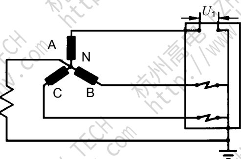
Figure 25a – Circuit préféré
