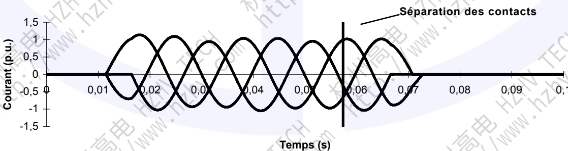
Figure 30 – Représentation graphique des trois coupures valables sur courants symétriques lors d'essais effectués en triphasé pour un réseau à neutre mis directement à la terre (facteur de premier pôle 1,3)
