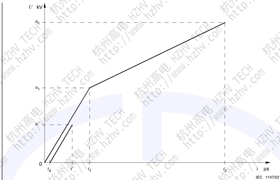
Figure 10 – Représentation d'une TTR spécifiée à quatre paramètres et d'un segment de droite définissant un retard pour les séquences d'essais T100, T 60, de défaut proche en ligne et en discordance de phases
