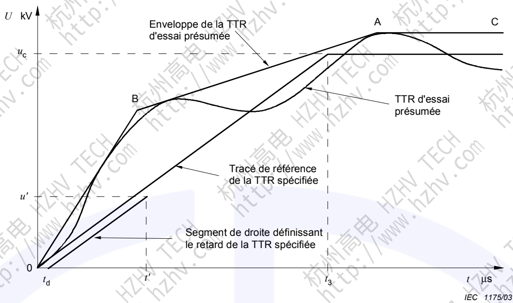
Figure 41 – Exemple d'une TTR d'essai présumée comportant une enveloppe à quatre paramètres répondant aux conditions imposées pour l'essai de type – Cas de la TTR spécifiée comportant un tracé de référence à deux paramètres
