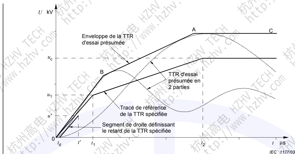
Figure 43 – Exemple d'ondes de TTR d'essai présumée et de l'enveloppe de l'ensemble pour des essais en deux parties
