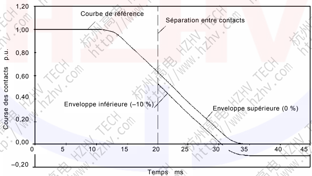
Figure 23d – Caractéristique de déplacement mécanique de référence (courbe idéalisée) avec l'enveloppe prescrite déplacée totalement vers le haut par rapport à la courbe de référence (+0 %, -10 %), dans cet exemple la séparation des contacts à lieu à t = 20 ms
