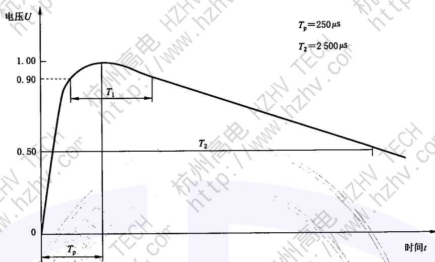
图2 操作冲击电压波
