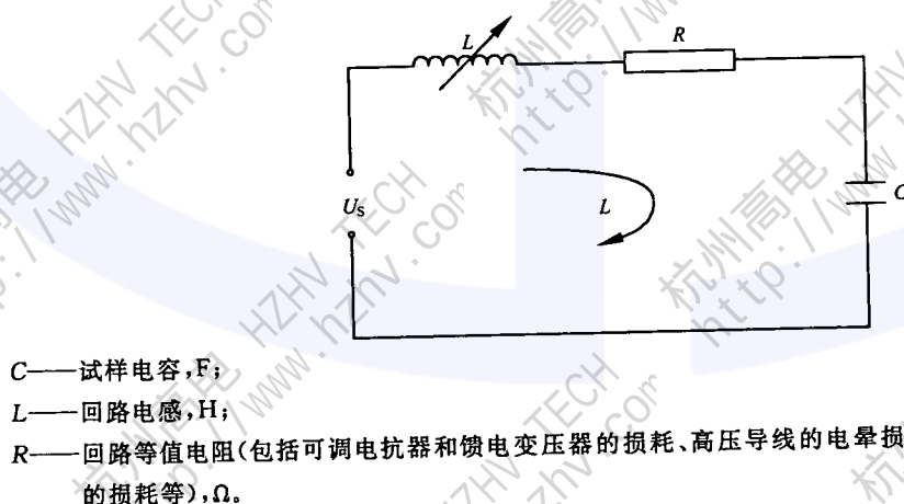
图 A.2 等值线路
