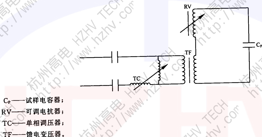
图 A.1 串联谐振试验回路
