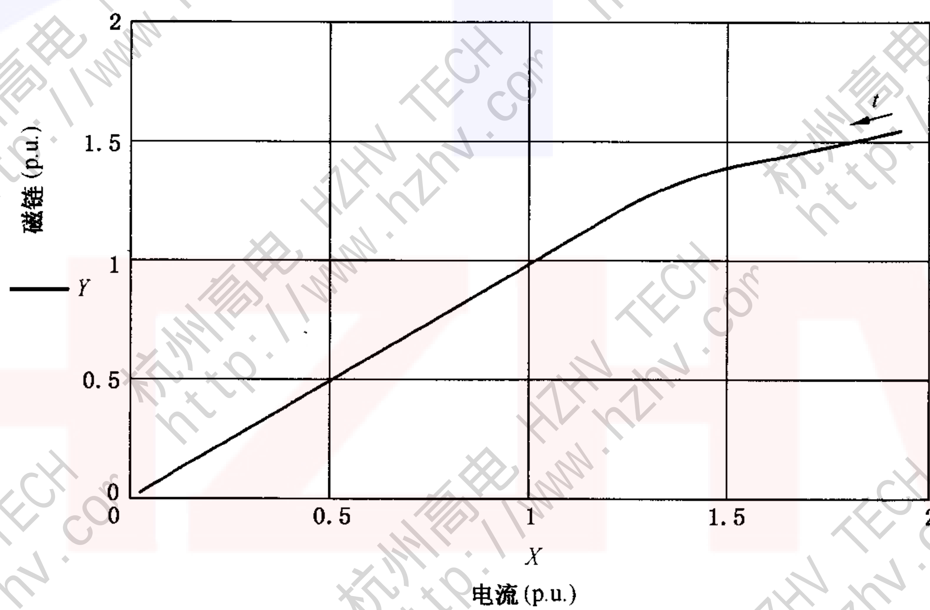
图 C.6 磁化特性
