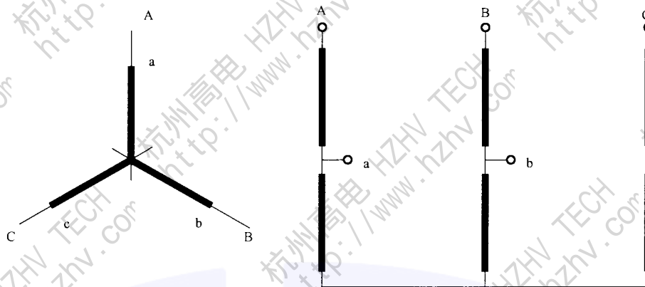
图 C.3 三相自耦变压器的联结组示例(联结组标号为 Ya0)
