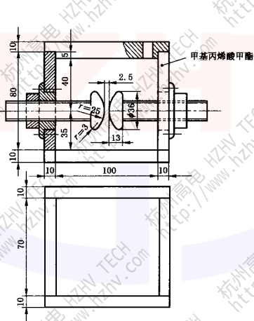
图 1 试样杯和球形电极
