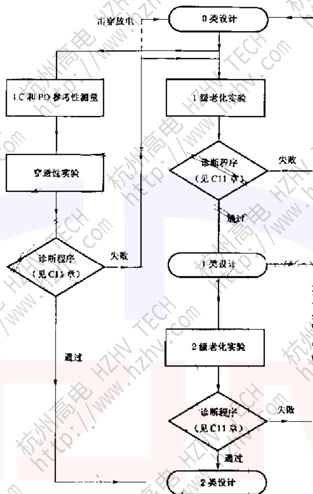
图 C.1 分类程序流程图
