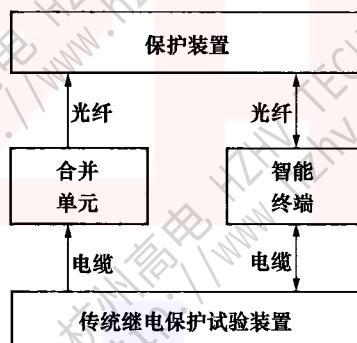
图 3 继电保护测试系统 3
