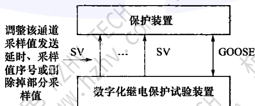
图 13 采样值传输异常测试接线图
