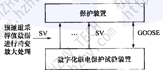
图 11 采样值数据畸变测试接线图
