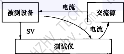
图 D.6 电流测试图
