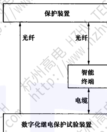
图 2 继电保护测试系统 2
