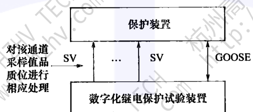
图 10 采样值数据标识异常测试接线图
