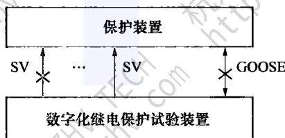
图 12 通信断续测试接线图
