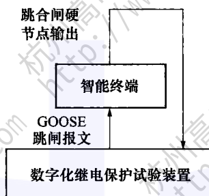
图 15 智能终端动作时间测试接线图
