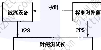
图 D.3 定时误差测试图
