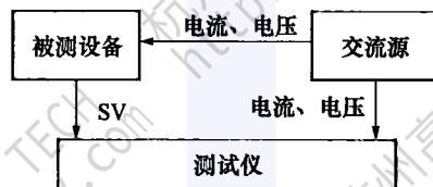
图 D.4 额定延时测试图
