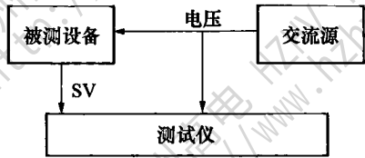
图 D.7 电压测试图
