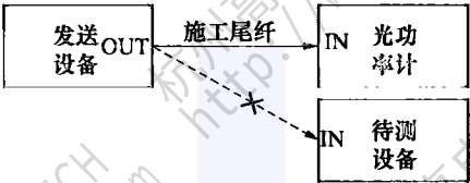
图 5 光纤端口接收功率检验方法
