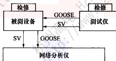
图 D.8 检修测试图
