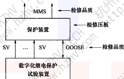
图 14 GOOSE 检修状态测试接线图
