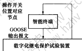
图 16 智能终端传送位置信号测试接线图
