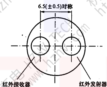
图 3 光口正视图
