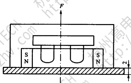
a) 吸力, 磁力线方向: N 极轴线指向多功能电能表 b) 尺寸: 内径 d_i=13\text{mm}\pm 1\text{mm} , 外径 d_o=28\text{mm} (最小值)
