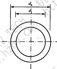
a) 吸力, 磁力线方向: N 极轴线指向多功能电能表 b) 尺寸: 内径 d_i=13\text{mm}\pm 1\text{mm} , 外径 d_o=28\text{mm} (最小值)
